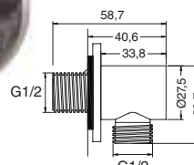
30057 Rociador lateral cuadrado antical Square side spray, anti-scale
